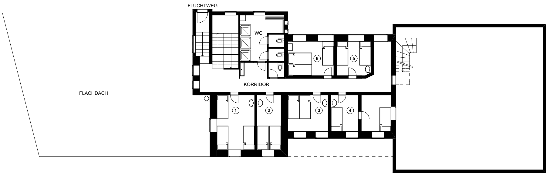
ERDGESCHOSS MST. 1:200
