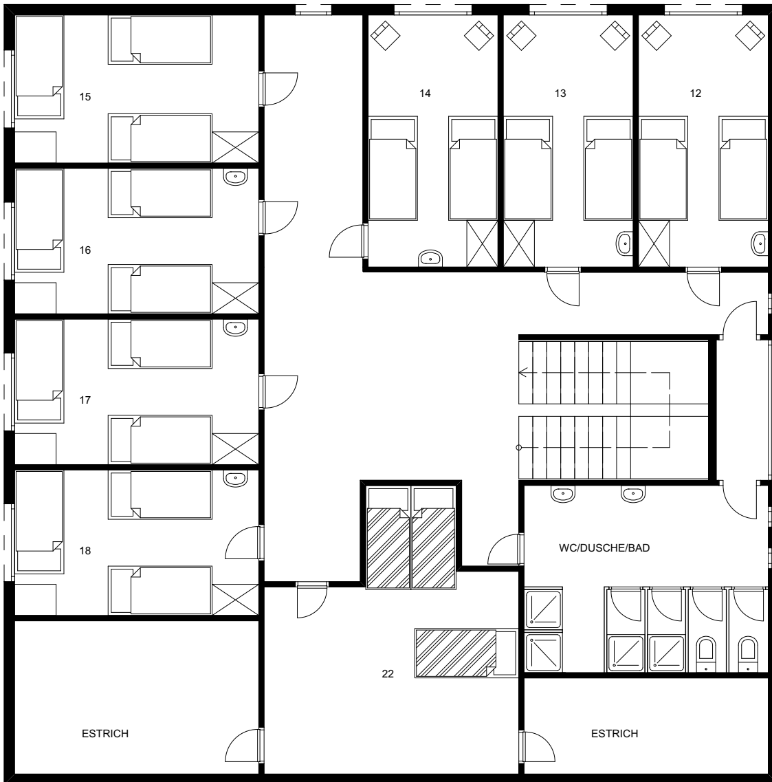
2.OBERGESCHOSS MST. 1:200
